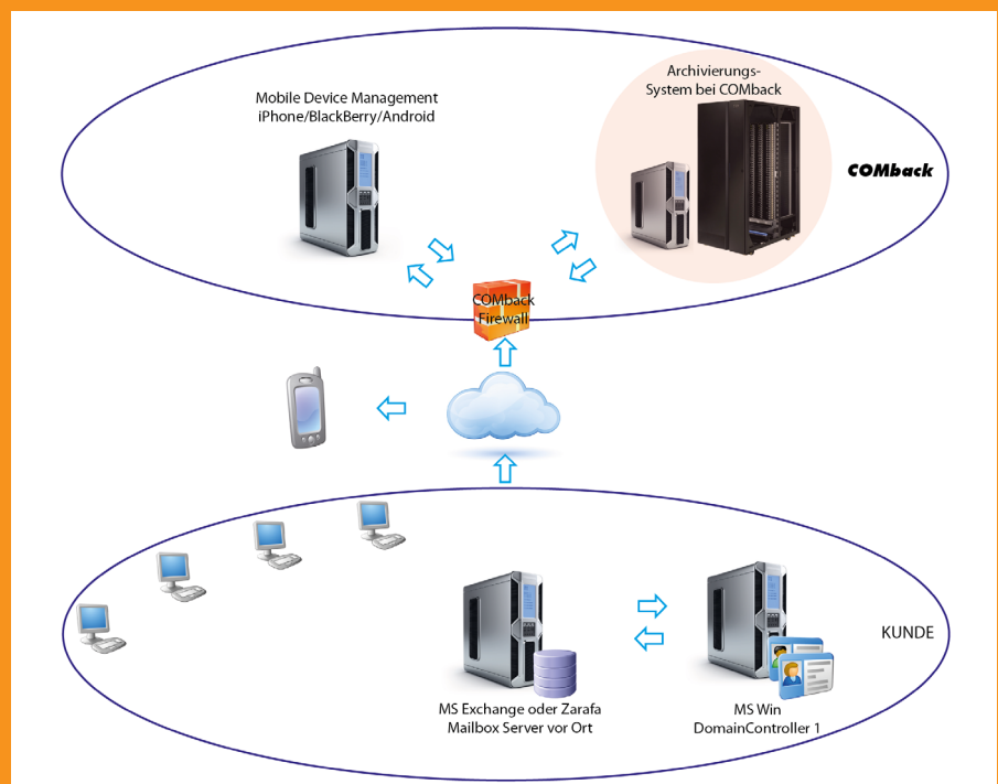
Bild 2: Auslagerung der Archivdaten ins COMback-Rechenzentrum + gehostete Betreuung der Mobilgeräte durch MDM-Server
